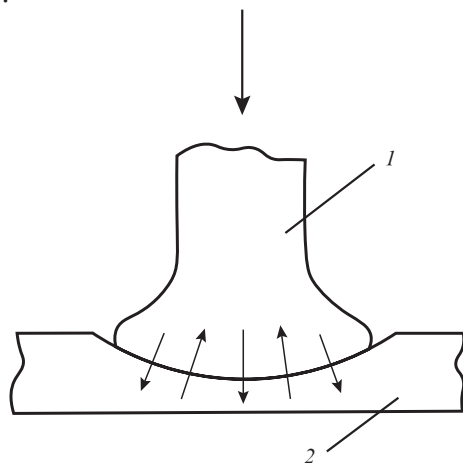
Расми 84. Тарзи иҷрои сикказанӣ: 1 - фӯлодқалам; 2 - масолеҳ.
