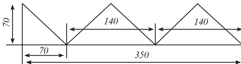
Расми 92. Тарзи тақсими масолеҳ барои мустаҳкамкунии бозуи болоӣ
