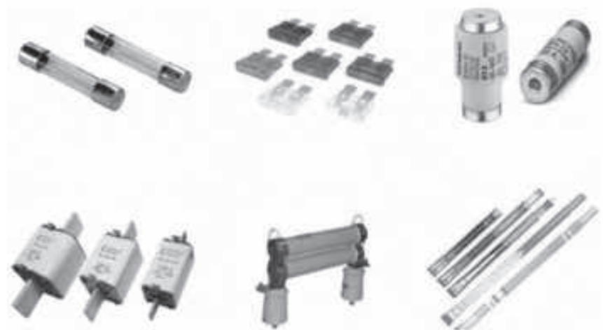
Расми 44. Намудҳои муҳофизии зудғудоз
