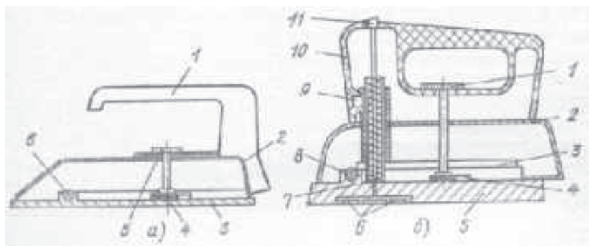
Расми 52. Дарзмол. а) танзимкунандаи ҳарорат; б) намкунанда: 1 – тугмачаи танзимкунандаи ҳарорат; 2 – асос; 3 – зарфи махсус; 4 – танзимкунандаи биметаллии ҳарорат; 5 – таг; 6 – роҳҳои обгузар; 7 – клапан; 8 – ТЭН; 9 – сӯроҳӣ барои обпуркунӣ; 10 – даста; 11 – тугмачаи обпошӣ.
