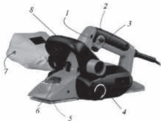
Расми 61. Сохти рандаи барқӣ: 1 – тугмаи қатъ кардани фаъолият; 2, 8 – дастакҳо; 3 – тугмаи пайвасткунӣ ва хомӯшкунӣ; 4 – сӯроҳии пара-ха бароранда, 5 – плитаи такякунӣ; 6 – асбоби назорати чуқуриши ранда; 7 – халтаи парахагундор.
