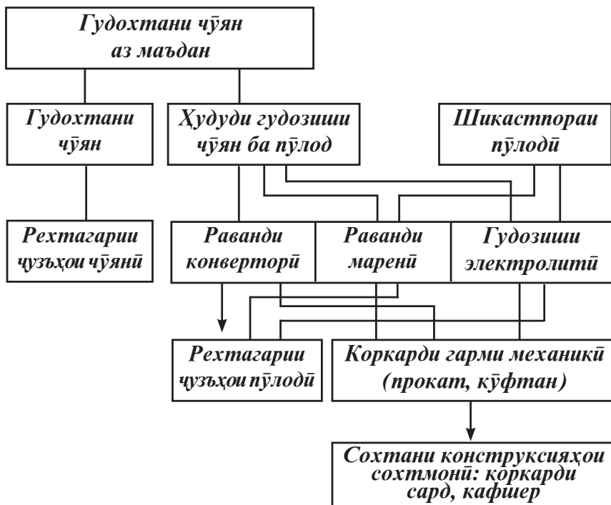
Расми 3. Асосҳои технологиҳои истеҳсоли пӯлод
