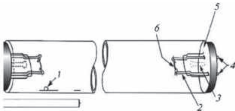
Расми 37. Чароғи люминесцентӣ: 1 – симоб; 2 – пойи шишаи хаттори барқӣ; 3 – найи пур аз газ; 4 – нуқтаи хат; 5 – панели маг; 6 – катоди эмиттериш.
