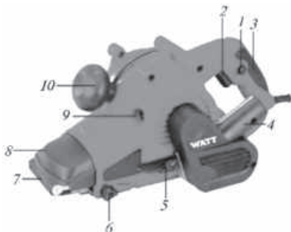
Расми 63. Сохти мошини суфтакунӣ: 1 – тугмаи блоккунӣ; 2 – тугмаи огози кор; 3 – даста; 4 – чангкашак; 5 – сорбити маҳкамкунандаи сарпӯши пеш; 6 – винти росткунӣ; 7 – тасмаи суфтакунӣ; 8 – сарпӯши пеш; 9 – қисми ҷимояи ҷӯткаҳои карбон; 10 – дастаки пеш.
