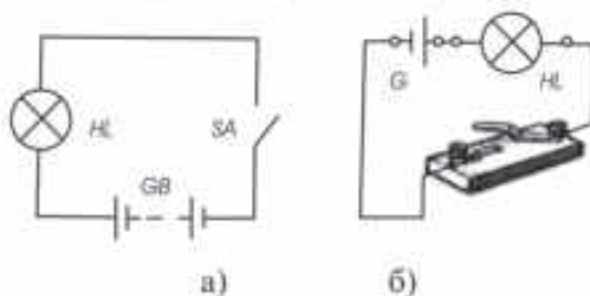
Расми 33. а) Нақшаи принципиалии занчири одӣ.
