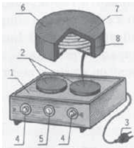
Расми 54. Манқали барқӣ: 1 – бадана; 2 – гармжунак; 3 – ноқили барқӣ бо вилка; 4 – калиди танзимкунандаи ҳарорат; 5 – чарогак; 6 – асоси чӯянӣ; 7 – унсури гармидиҳандаи найчагӣ; 8-қабати гарминигоҳдоранда
