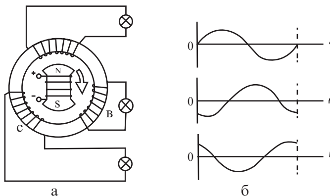
Расми 47. Ҳосилишавии ҷараёни барқӣ сефазагӣ
