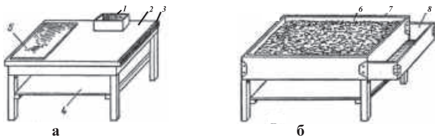
Расми 82. Қойи кори сикказан: а) мизи корӣ, б) қуттӣ бо қум. 1. қуттӣ барои асбобҳо; 2. рӯйи миз; 3. кунҷаки пӯлодӣ; 4. раф барои халта бо қум; 5. лавҳаи пӯлодӣ; 6. қум; 7. тарафҳои қуттӣ; 8. қой барои асбобҳо.
