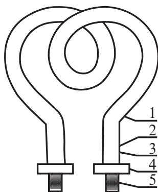
Расми 51. Унсури гармидиҳанда: 1 – найчаи металлӣ; 2 – спиралӣ гармкунанда; 3 – реҗи кварсӣ; 4 – эмали махсус; 5 – штилкаи пайвандӣ.
